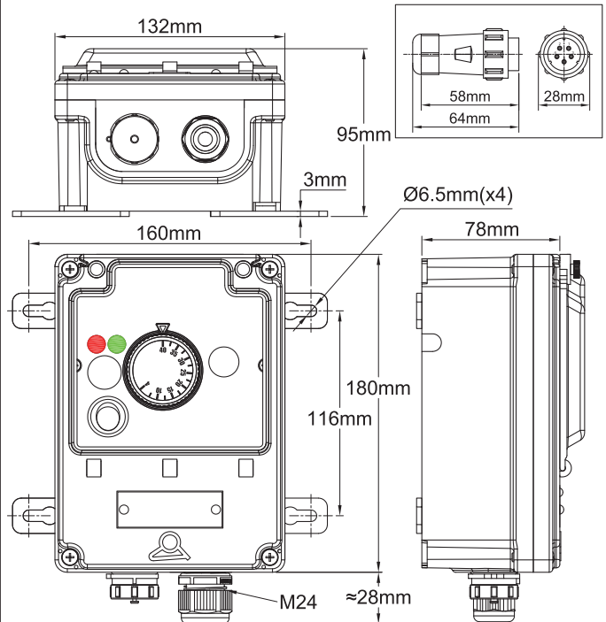
Modelo con un conector de 5 vías y una glándula de cable M24: Y8WR-Y
